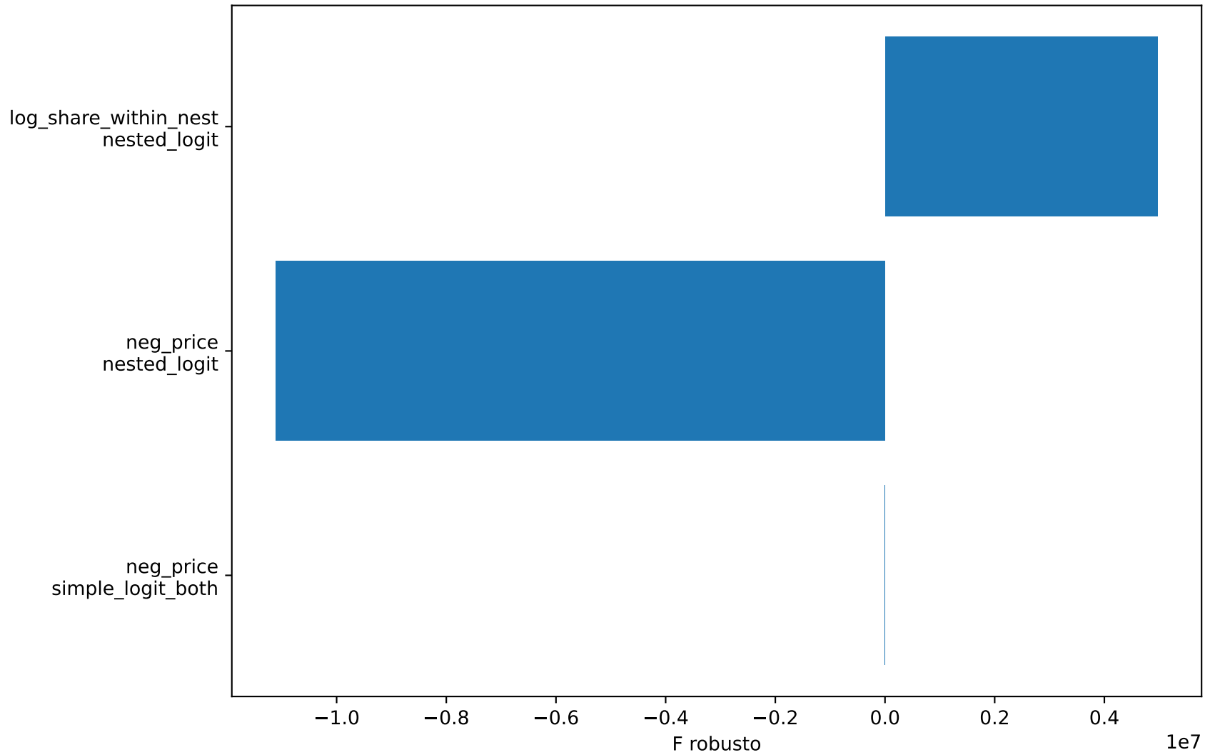
F/Wald-F robusto do primeiro estágio
